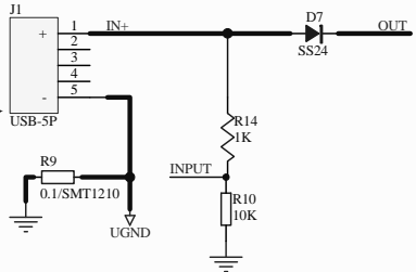
USB插入检测部分
