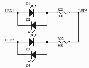
电量指示部分
