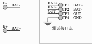
电池接口与测试点
