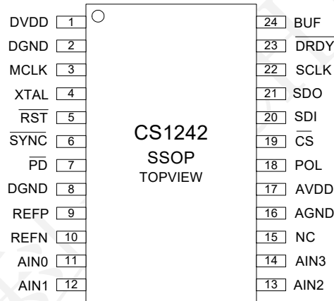
图 3 CS1242_SSOP24 芯片引脚图
