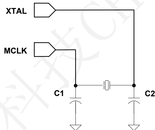
图 6 外部晶振连接图
