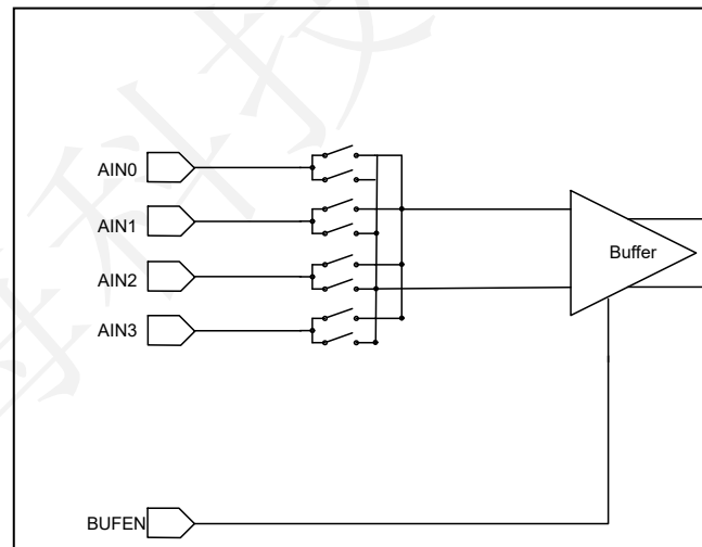
图 5 多路输入选择原理框图
