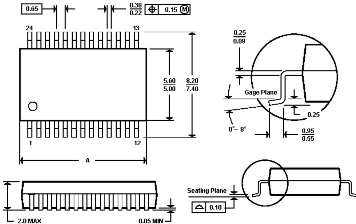
图 8 SSOP24 封装轮廓图
