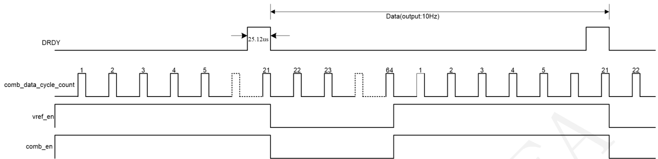
图 3.6 CS1251 低功耗工作示意图
