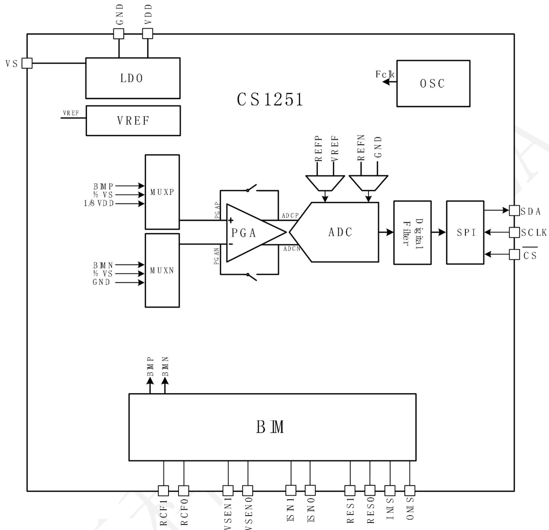
图 1.1 CS1251 原理框图
