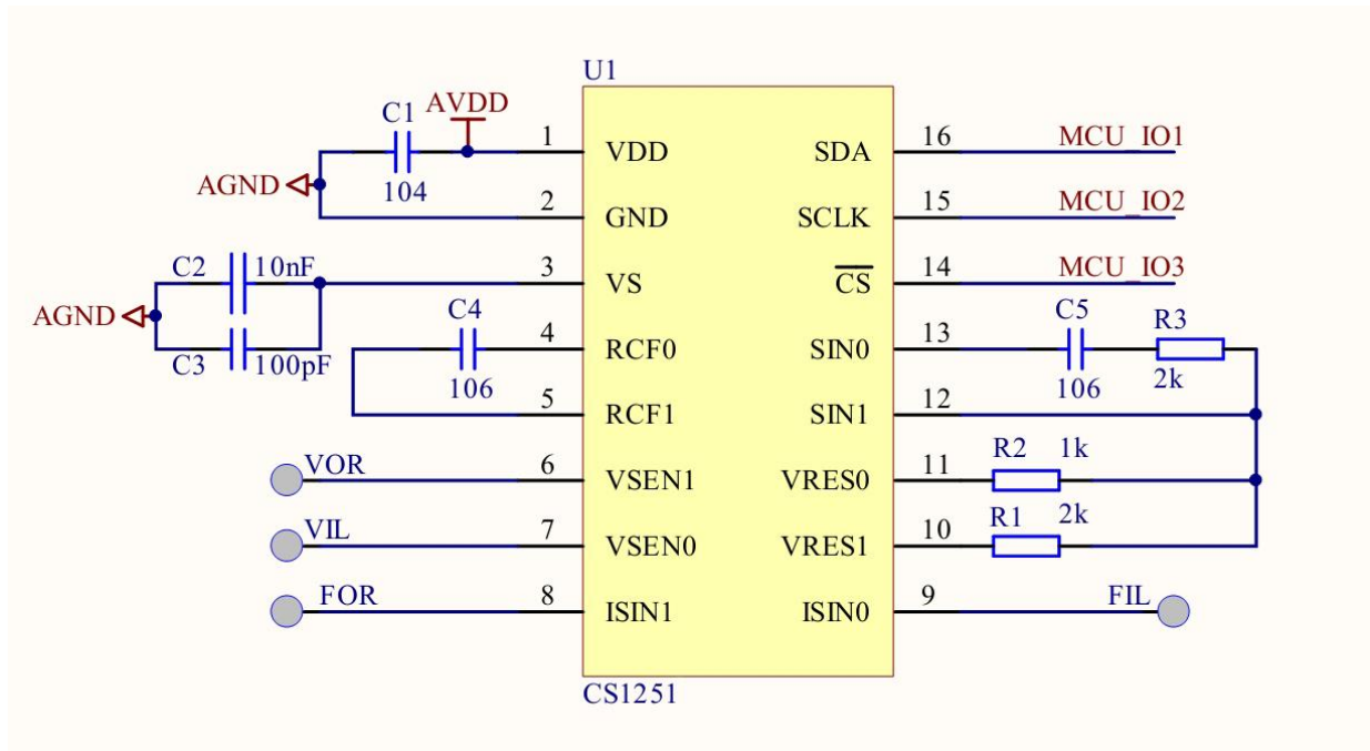
图 1.3 CS1251 典型应用电路
