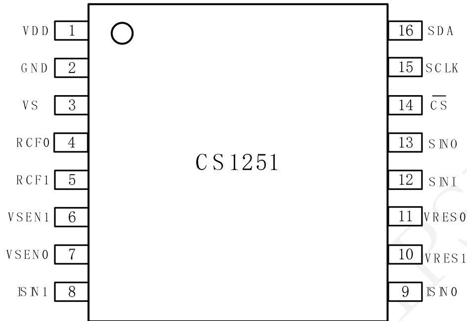
图 1.2 CS1251 引脚图
