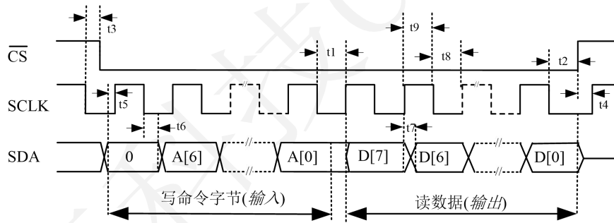
图 6.2 读操作时序 2(除 AD 值之外的寄存器)
