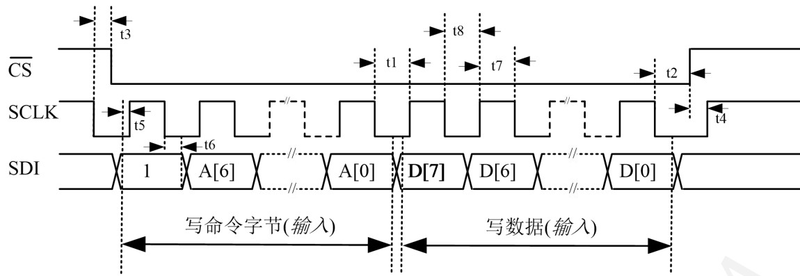
图 6.3 写操作时序
