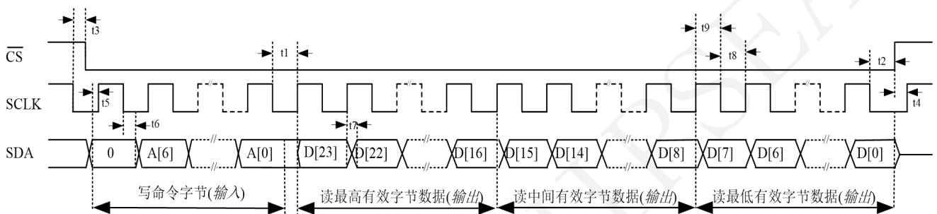
图 6.1 读操作时序 1(读 AD 值)
