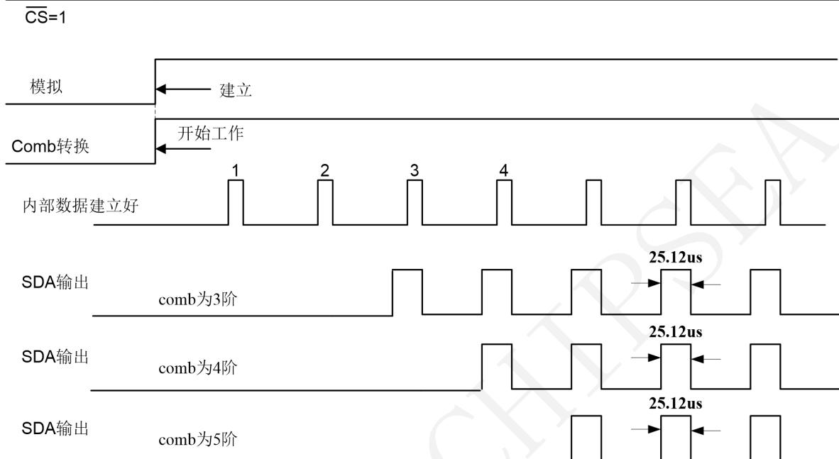
图 3.4 COMB 建立过程
