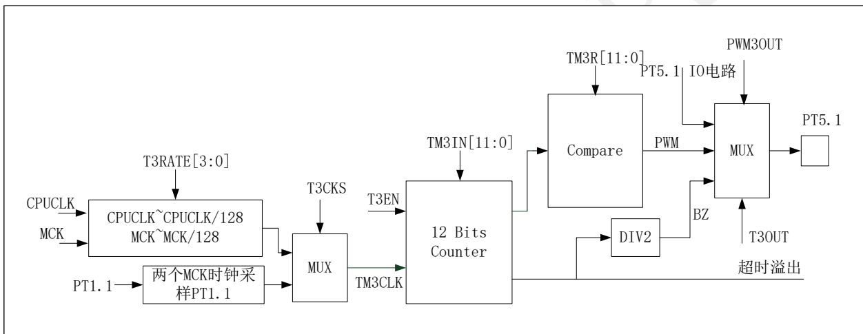
图19 定时/计数器 3 模块的功能框图
