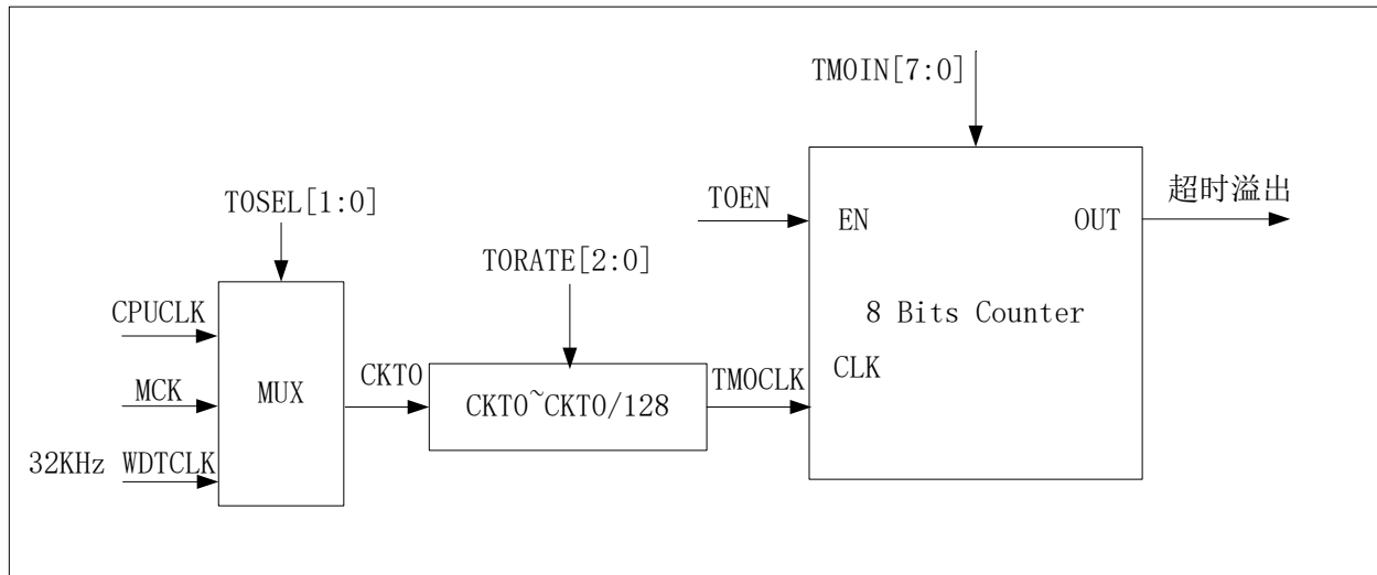
图13 定时器 0 功能框图
