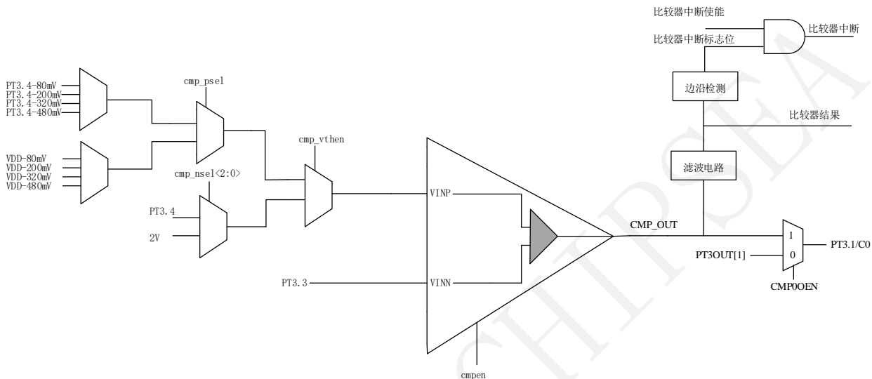
图25 模拟比较器框图
