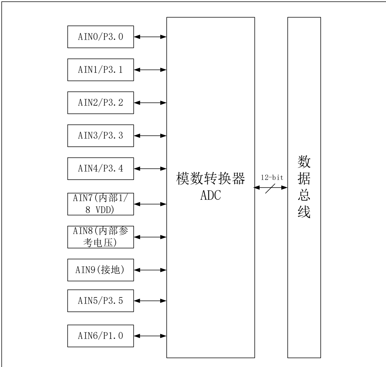
图24 模数转换器 ADC 功能框图
