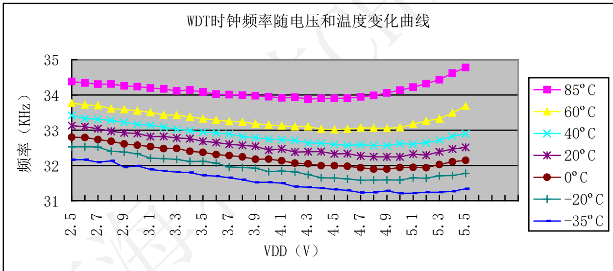
图32 WDT 频率的电压和温度特性
