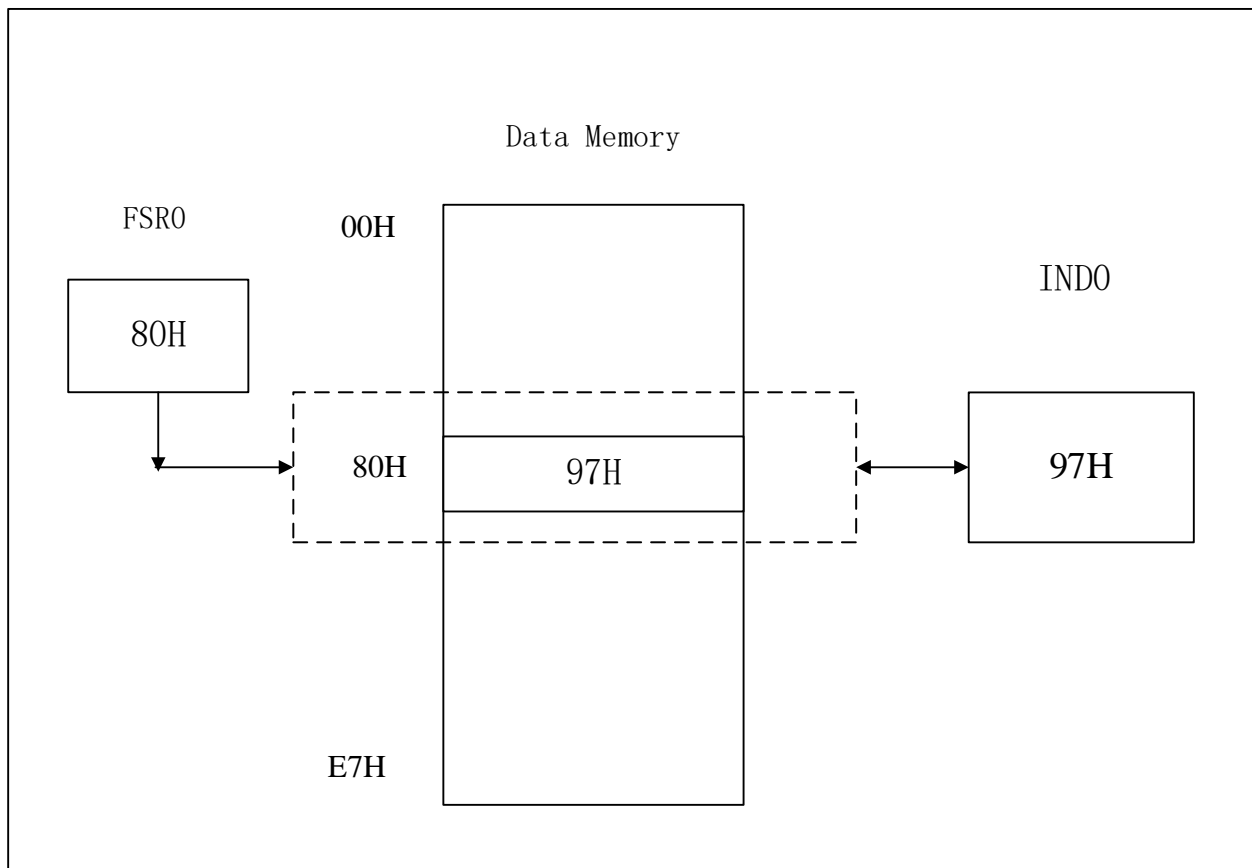
图7 间接地址访问
