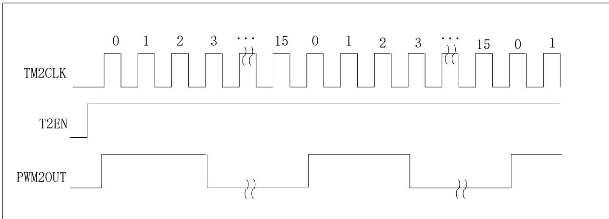
图18 TM2IN=0x0F ， TM2R=0x03 的 PWM2 波形输出
