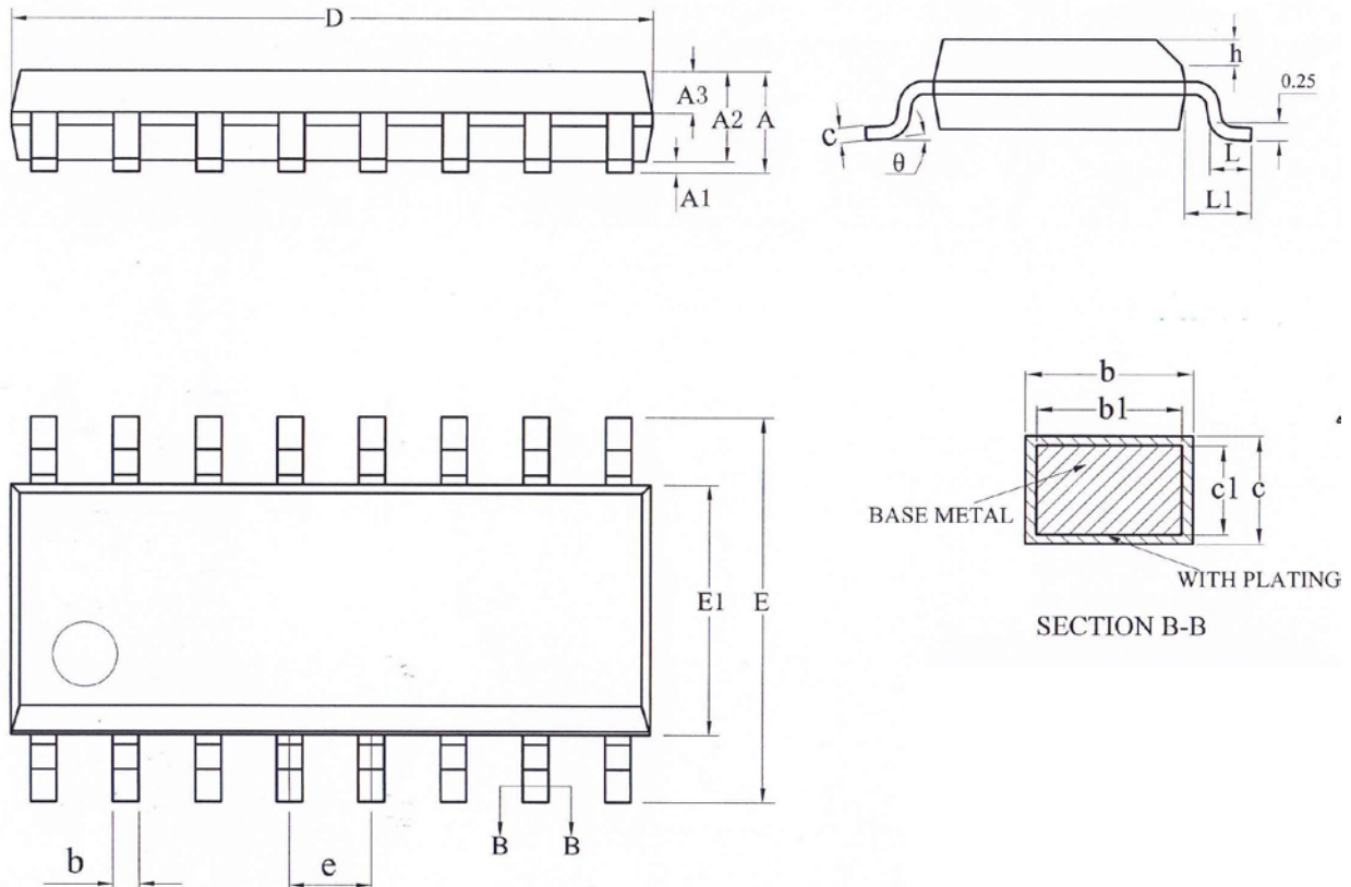
图41 SOP-16 封装框图
