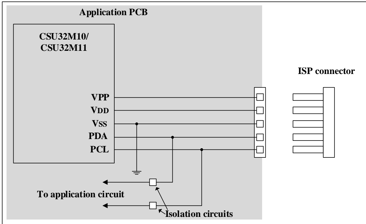
图27 烧录器接口图
