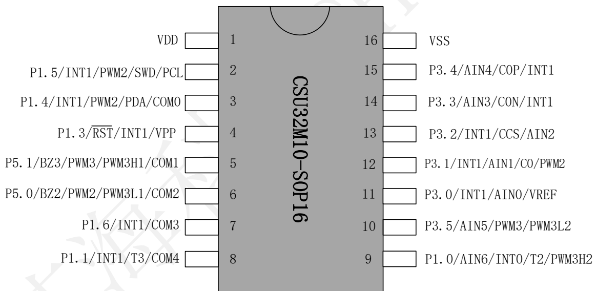
图2 SOP16-1 管脚图
