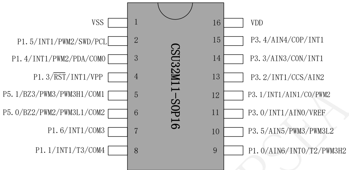
图3 SOP16-2 管脚图
