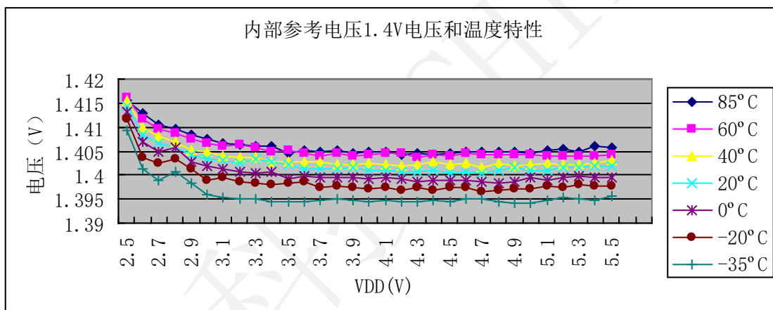
图36 内置参考电压 1.4V 电压和温度特性
