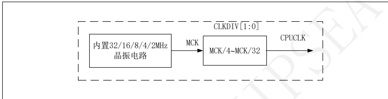
图8 CSU32M10/CSU32M11 振荡器状态框图
