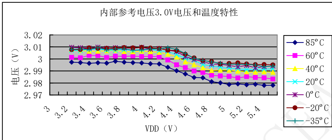
图38 内置参考电压 3.0V 电压和温度特性
