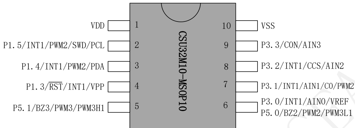
图1 MSOP10 管脚图
