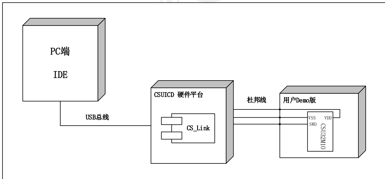
图26 在线调试系统框图
