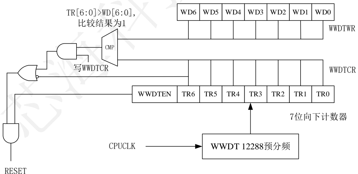
图15 WWDT 框图
