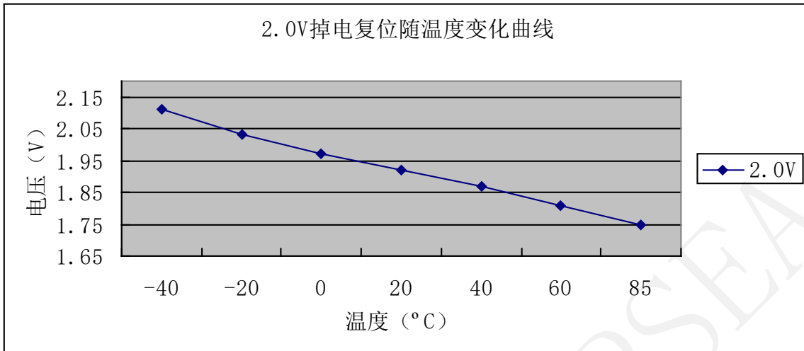
图33 2.0V 掉电复位温度特性
