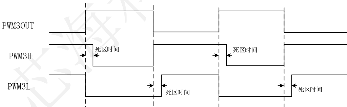
图23 PWM 输出取反后的互补 PWM 输出
