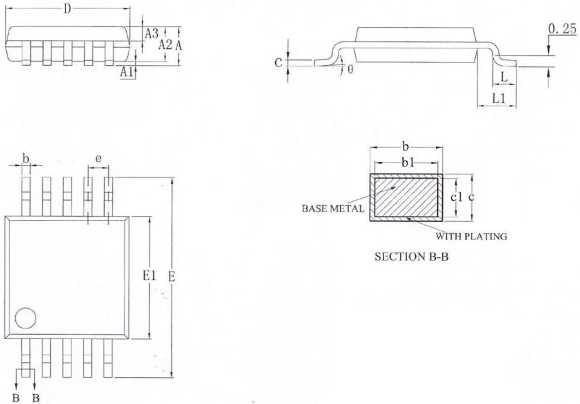
图40 MSOP-10 封装框图
