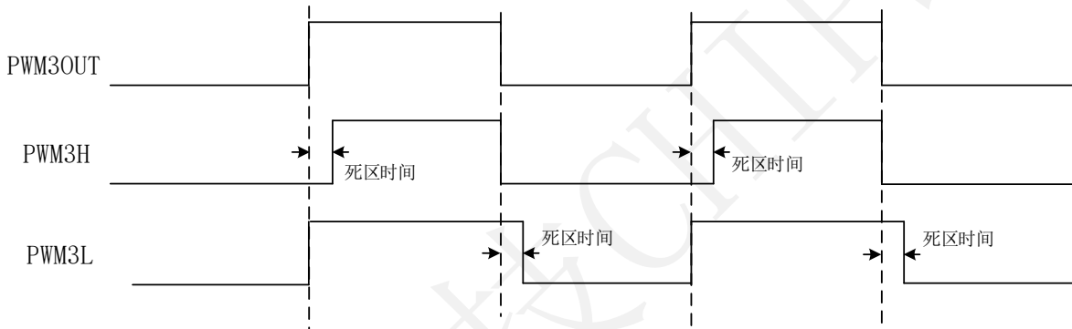
图22 互补式 PWM 输出波形
