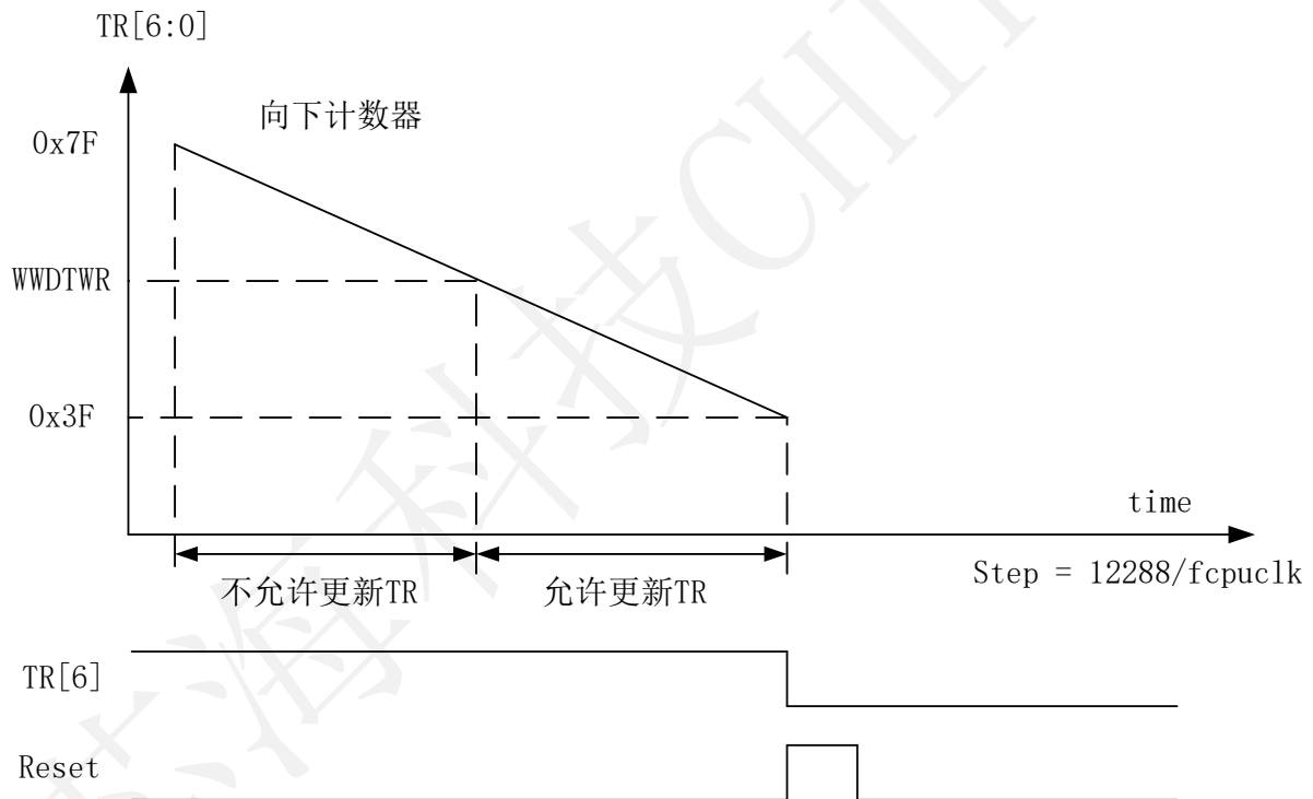
图16 WWDT 时序图
