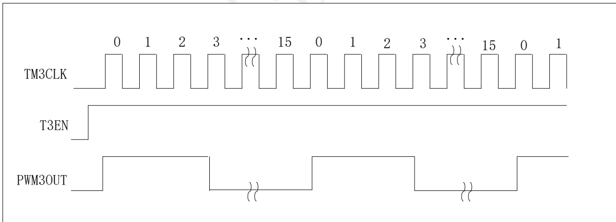
图20 TM3IN=0x0F ， TM3R=0x03 的 PWM3 波形输出
