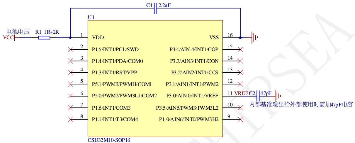
图28 参考电路
