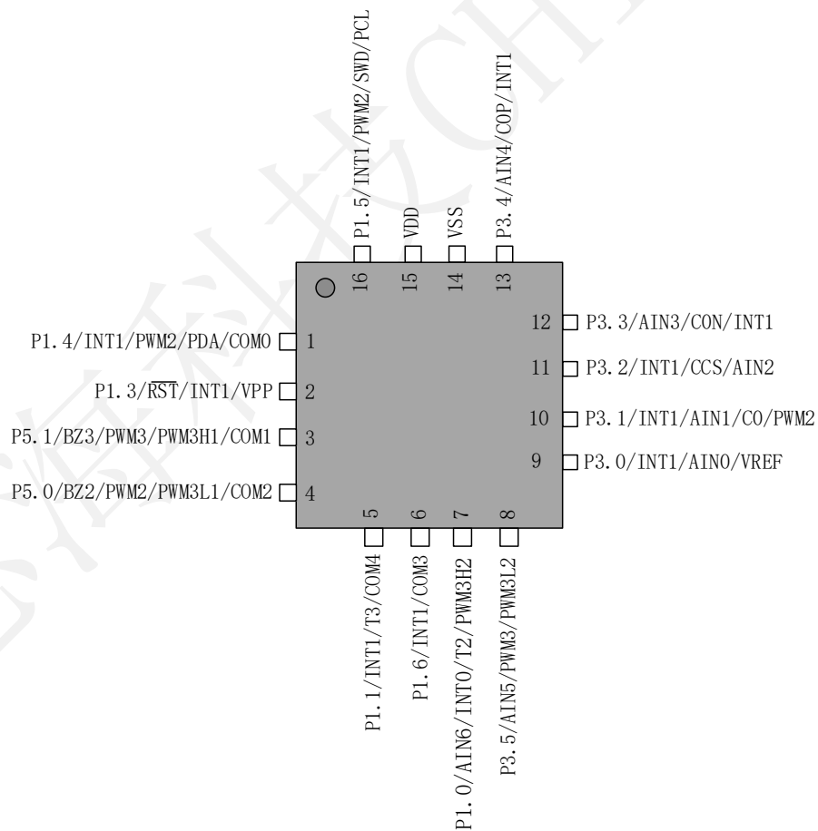
图4 QFN16 PIN 配置图
