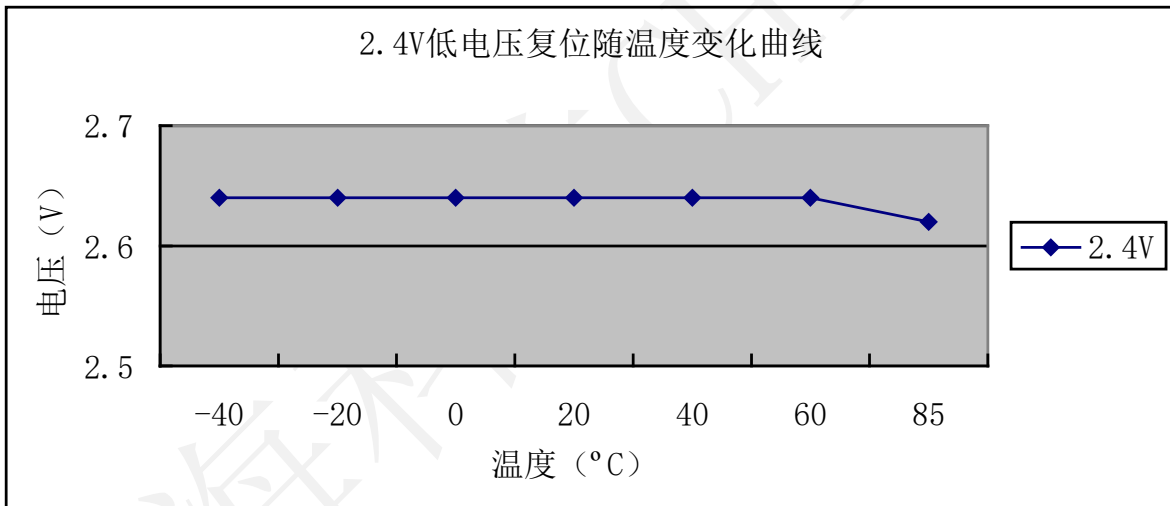
图34 2.4V 低电压复位温度特性
