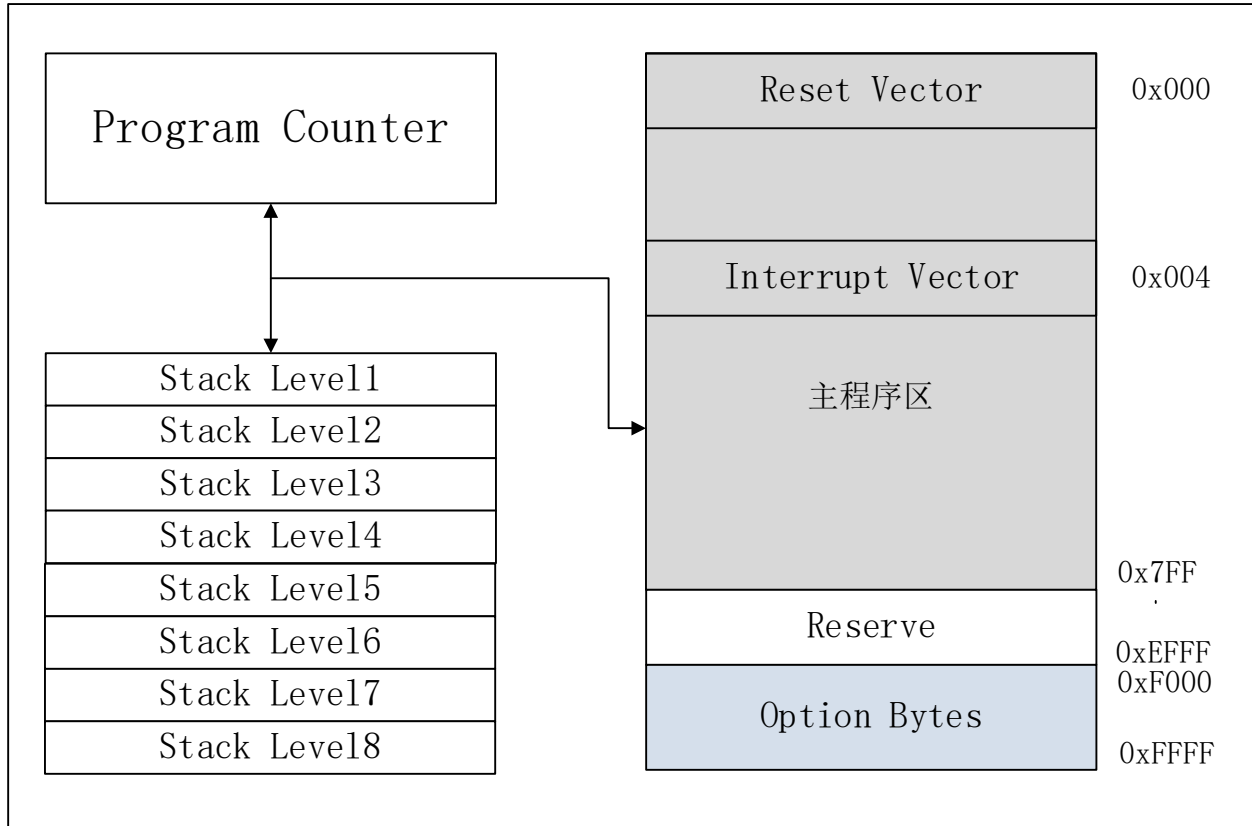
图6 程序存储器
