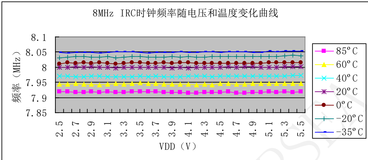
图31 8MHz RC 时钟频率的电压和温度特性
