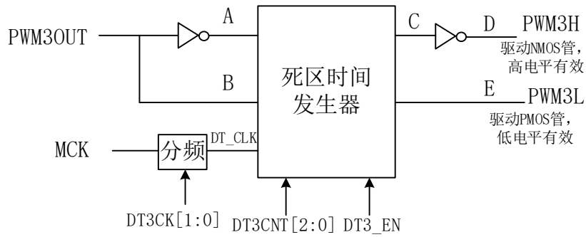
图21 互补式 PWM 输出方框图
