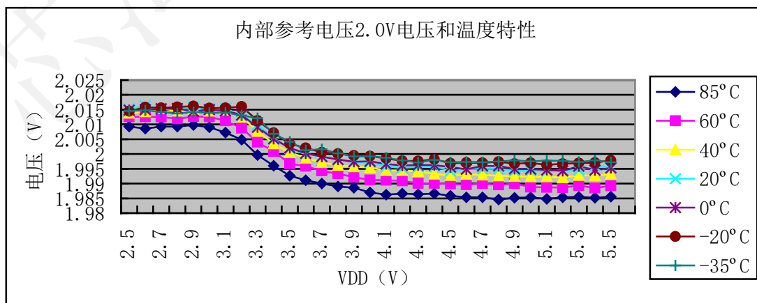
图37 内置参考电压 2.0V 电压和温度特性
