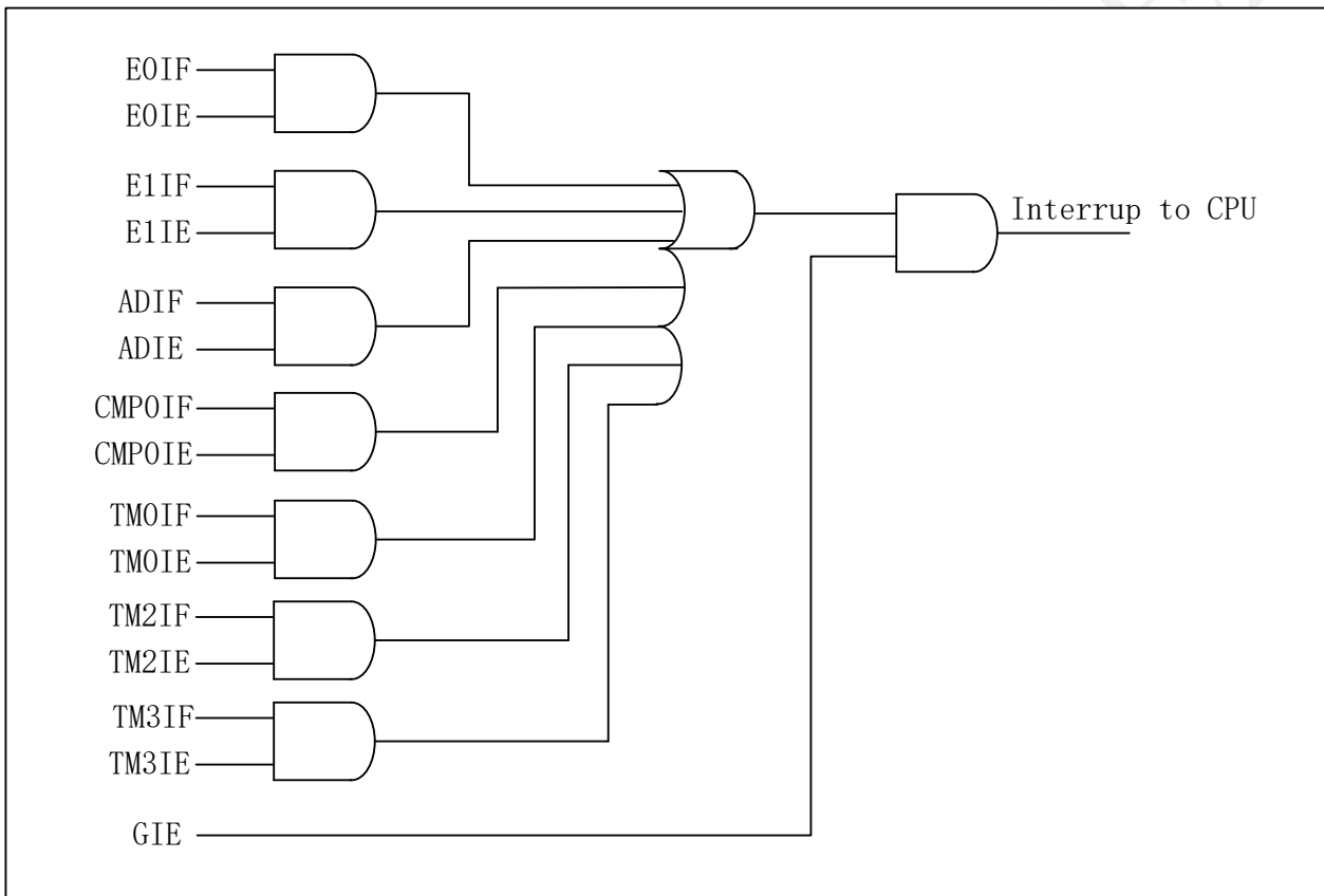
图12 中断逻辑
