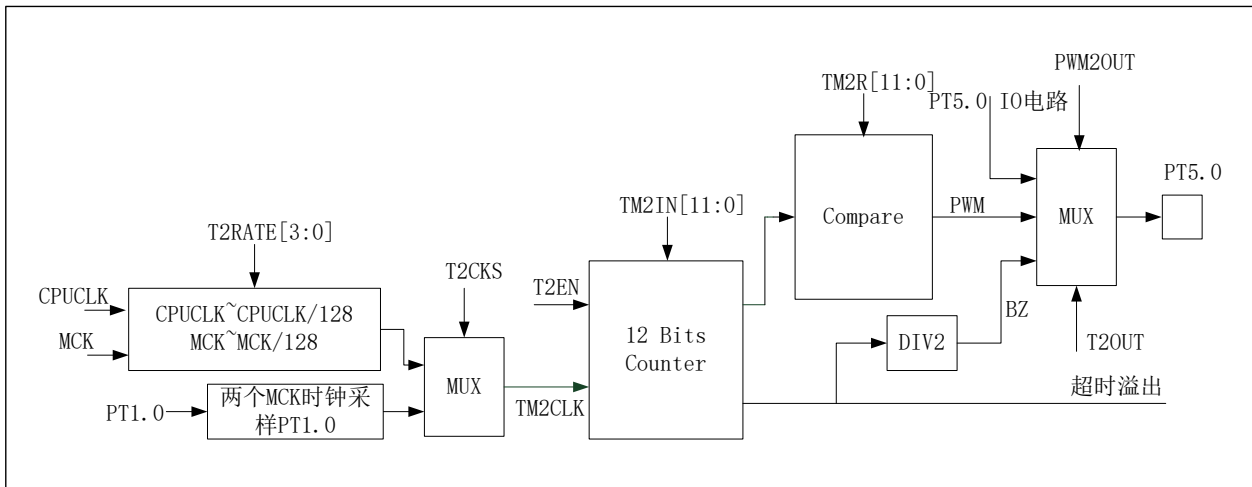
图17 定时/计数器 2 模块的功能框图
