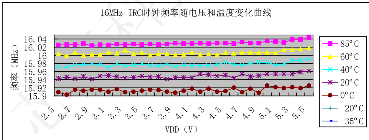
图30 16MHz RC 时钟频率的电压和温度特性
