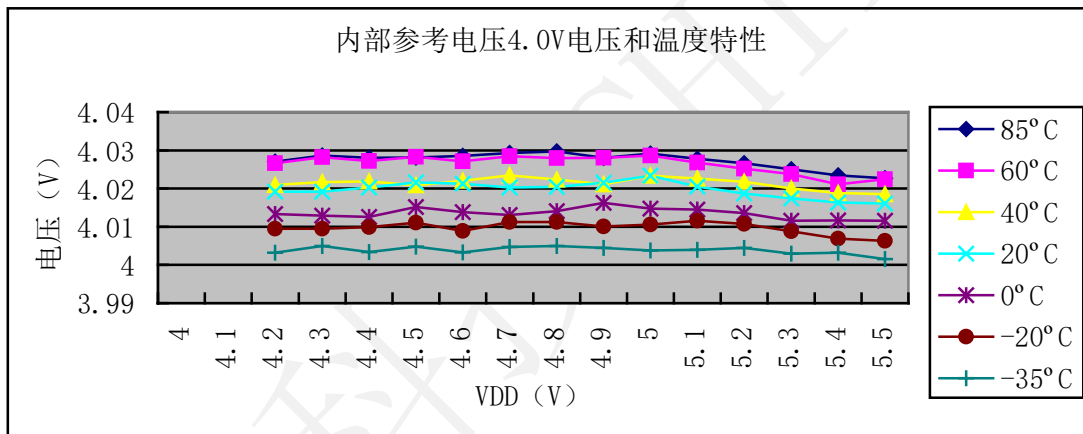
图39 内置参考电压 4.0V 电压和温度特性
