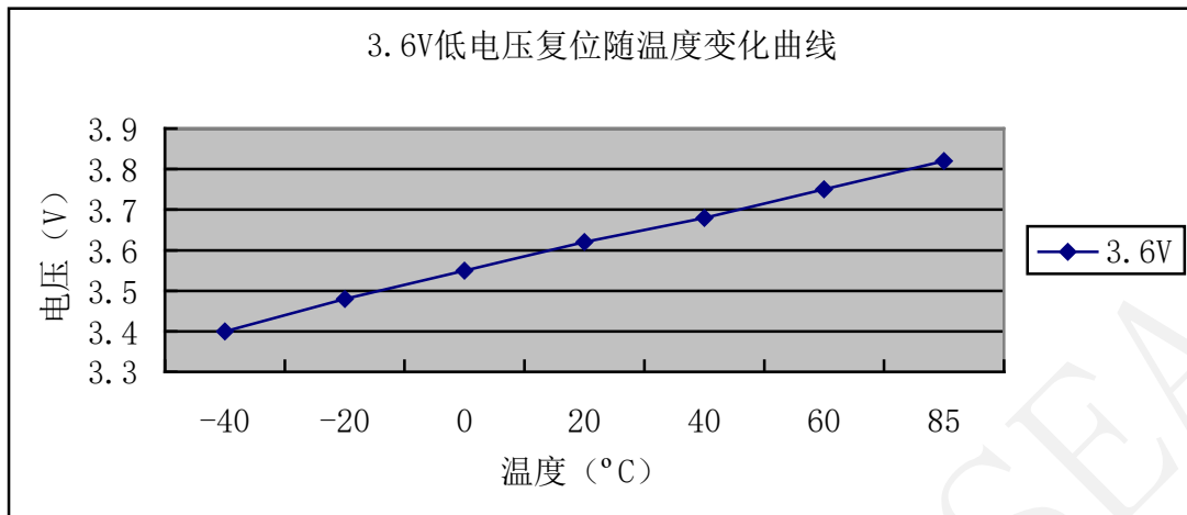
图35 3.6V 低电压复位温度特性
