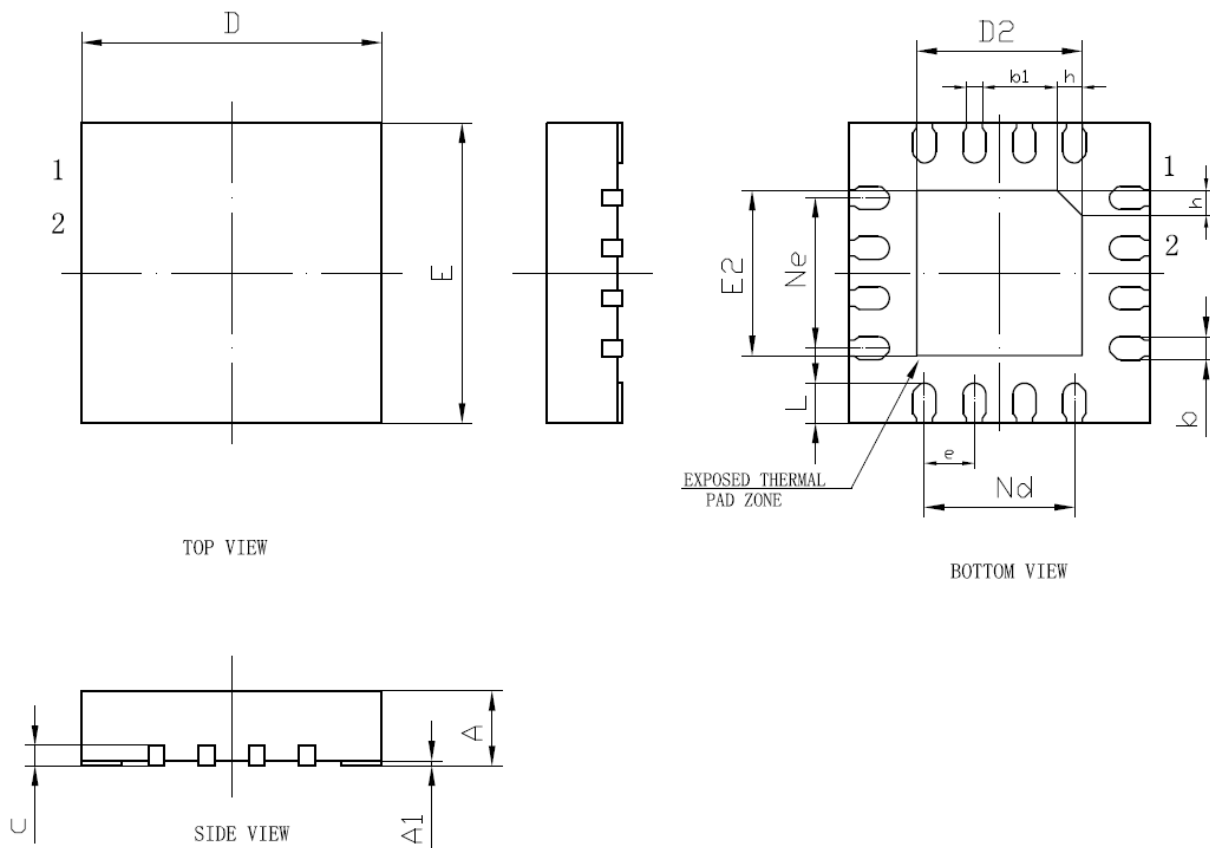
图42 QFN-16 封装框图
