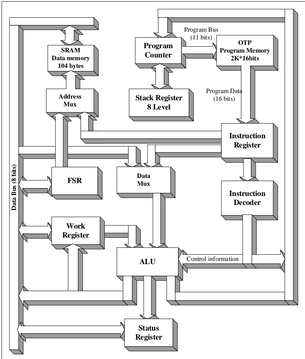
图5 CSU32M10/CSU32M11 CPU 核的功能模块图
