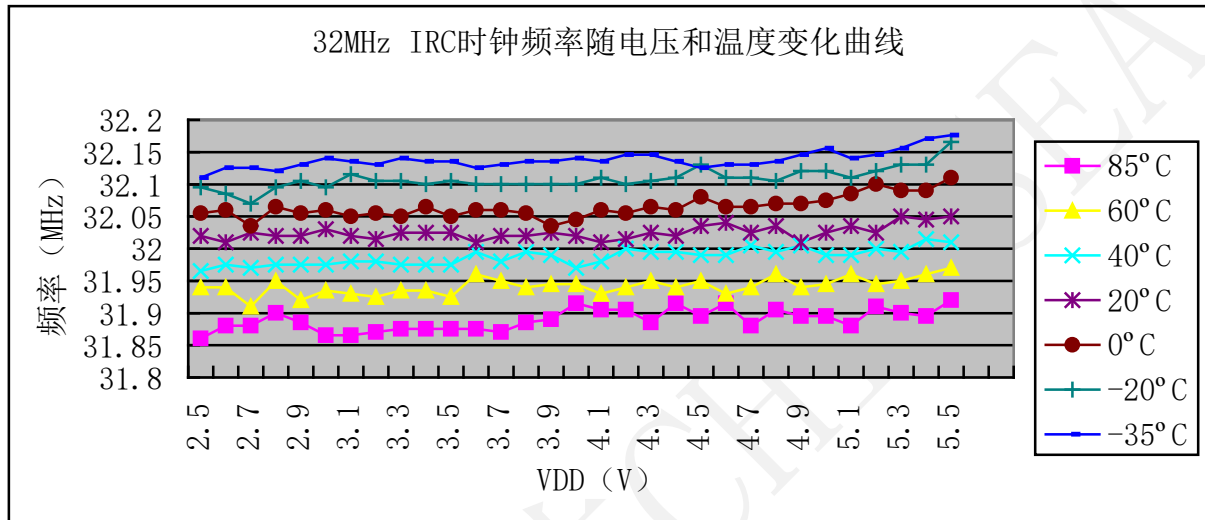
图29 32MHz RC 时钟频率的电压和温度特性
